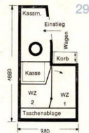
Modell COMBI- Zwei links 98
