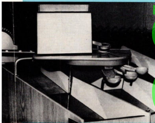
Rückgeldschleuse auch für NCR- und Hugin-Rückgeldautomaten. Das Rückgeld wird jeweils zu der geöffneten Warenzelle – in die hierfür vorgesehene Geldauffangschale geschleust.
