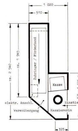
Maßzeichnung im Maßstab ca. 1:50. Wahlweise auch in anderen Abmessungen lieferbar.
