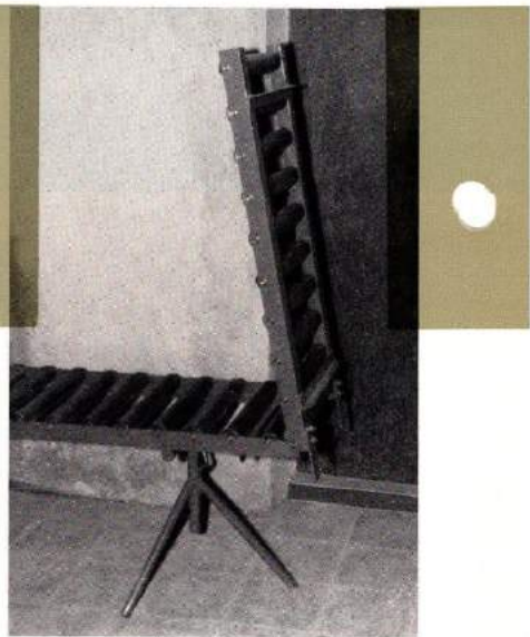
Rollenbahn klappbar als Durchgang und auch als Förderweiche lieferbar.
